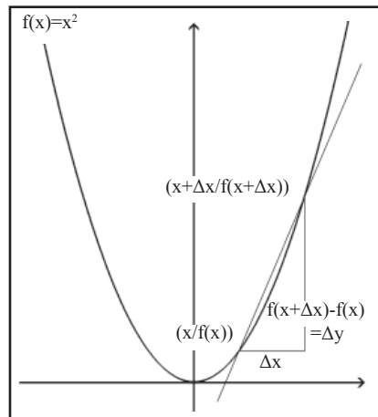
Fig.3: Berechnung der Steigung einer Sehne einer Parabel
